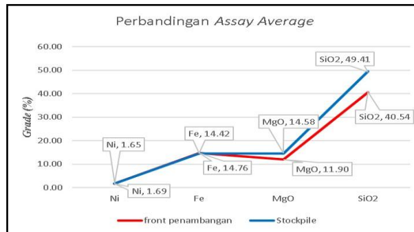
Gambar 1. Grafik perbandingan kadar Rata- Rata Endapan Nikel Laterit (Ni, Fe, MgO dan SiO 2 ).
