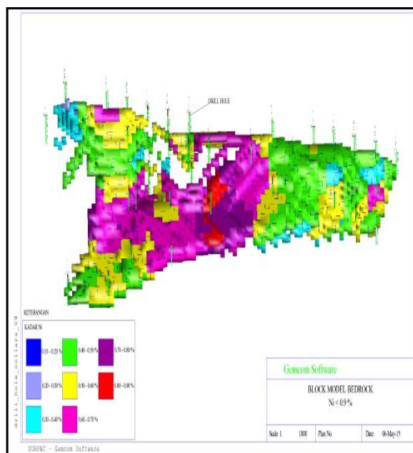
Gambar 12: Blok Model bedrock Ni <0,9%.
