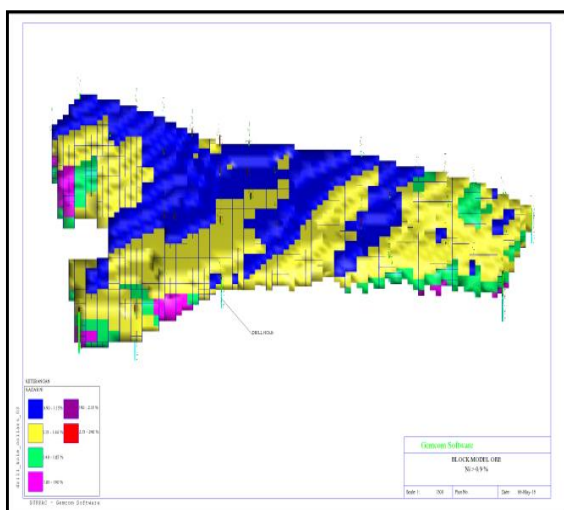
Gambar 11. Blok Model ore Ni >0,9%
